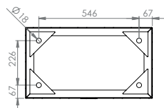
Base de cimentación SECCIÓN A-A
