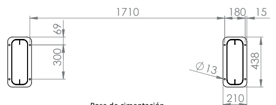
Base de cimentación Sección A-A
